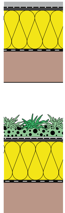
Oben: Flachdach mit Nutzschicht Unten: Flachdach mit Schutzschicht
